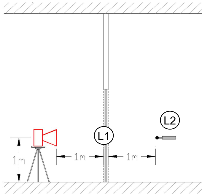
41. ábra: Beltéri ajtók hanggátlási tulajdonságainak vizsgálata a tűzjelzések hallhatóságával összefüggésben, Forrás: saját ábra
