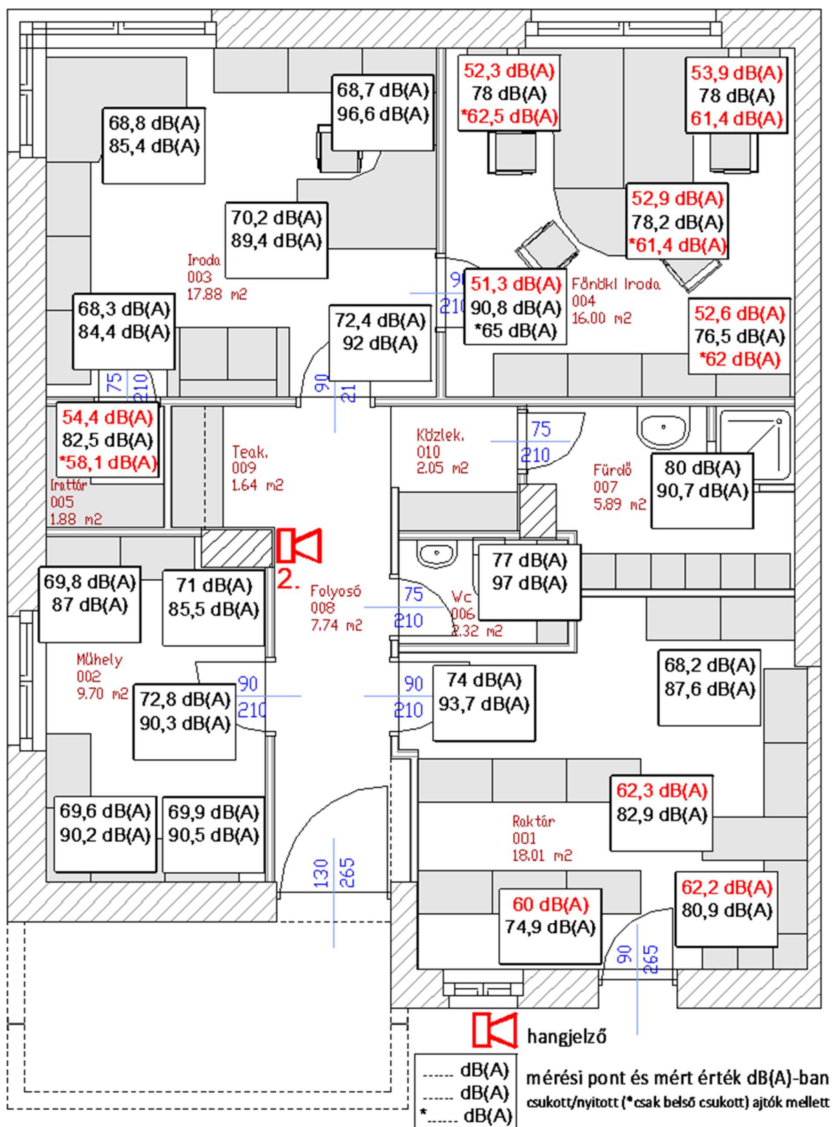
51. ábra: Mért hangnyomásszint értékek a 2. hangjelző pozícióban, csukott/nyitott és részben nyitott ajtók mellett, Forrás: saját
