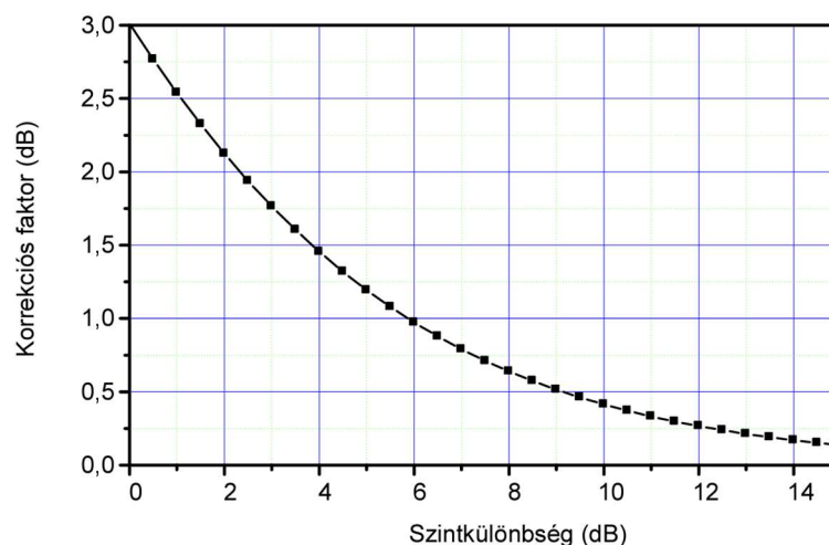
45. ábra: Két hangforrás egyidejű hatása esetén az eredő hangnyomásszint számolása [64]
