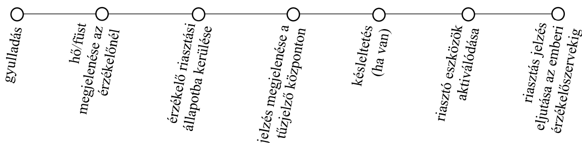
5. ábra: A tűzjelzés és riasztás időbeni folyamata, Forrás: saját ábra
