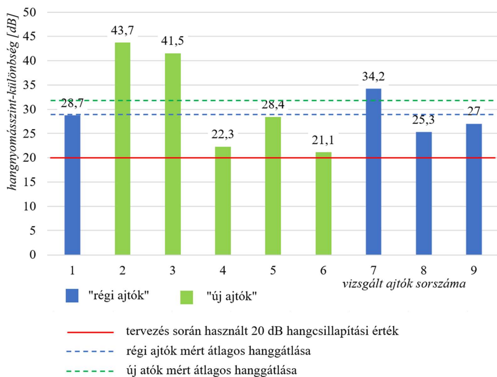
44. ábra: Beltéri ajtók hanggátló hatása a tűzjelzésre, forrás: saját mérések alapján
