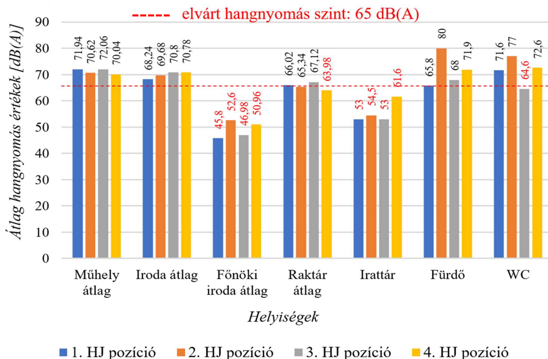
47. ábra: Különböző hangjelző pozíciók esetén mért hangnyomásszintek, Mérés 3), forrás: saját ábra
