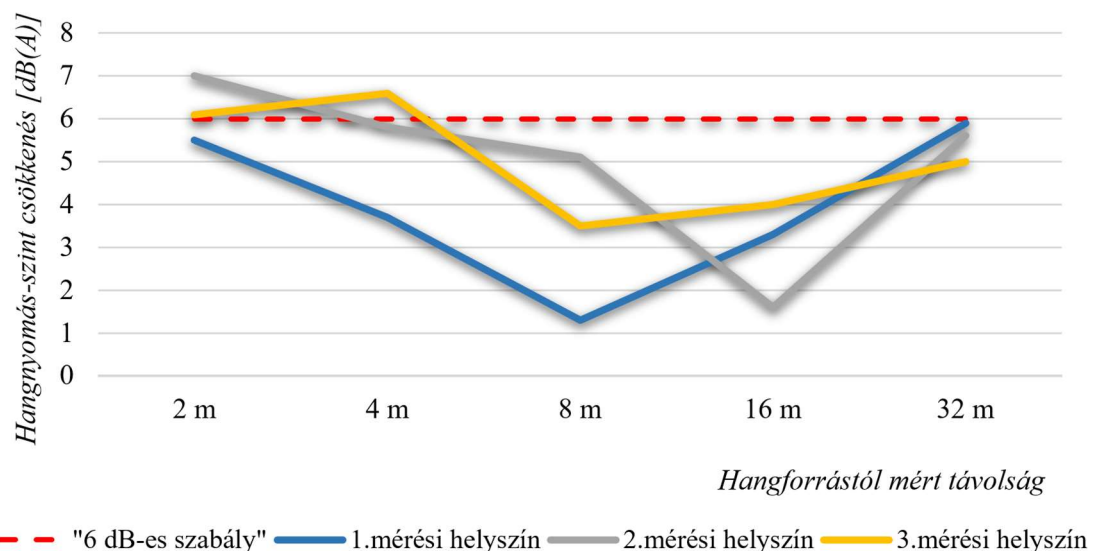
38. ábra: Mért hangnyomás-szint csökkenés a távolság függvényében, Forrás: saját ábra
