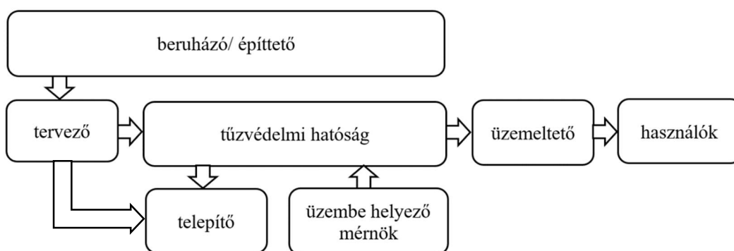
16. ábra: A tűzjelző berendezés létesítési folyamata és szereplői, Forrás: saját ábra
