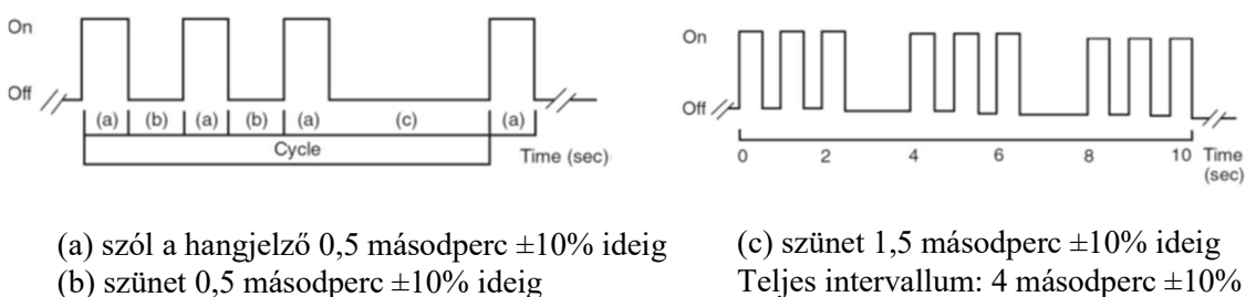
33. ábra: Standard 'Temporal-Three' tűz hangminta az NFPA 22 72 alapján, Forrás: [53]
