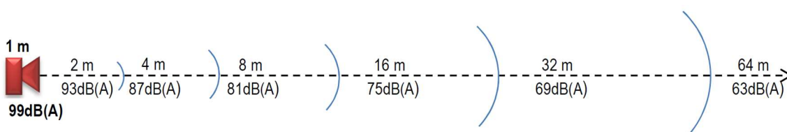
36. ábra: A „6-dB-es szabály” elvi értékei a hangforrástól távolodva, Forrás: [56]
