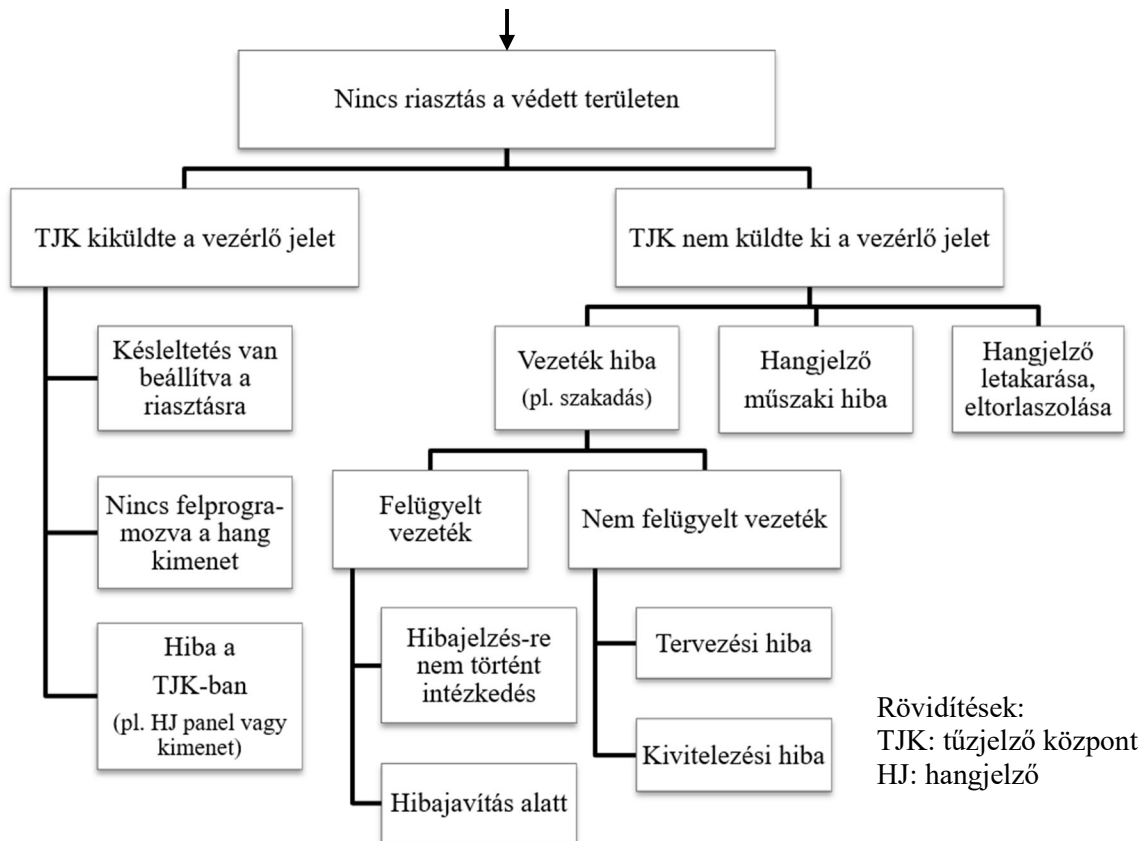
13. ábra: Logikai fa a riasztás meghiúsulásához vezető lehetséges okokról, Forrás: saját
