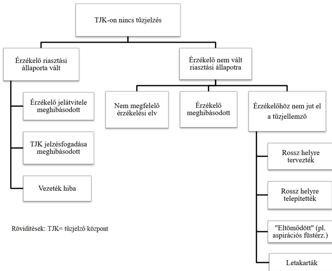
9. ábra: Logikai fa a tűzjelzés elmaradásához vezető okokról, Forrás: saját
