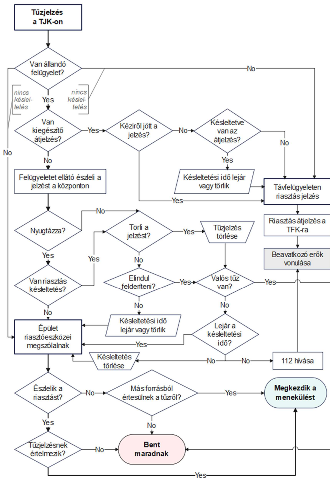
53. ábra: Tűzjelzést követő intézkedések folyamatábrája, Forrás: saját ábra
