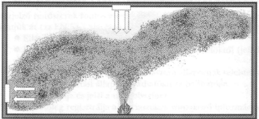
21. ábra: Légtechnika hatása az érzékelési időre, Forrás: [33]
