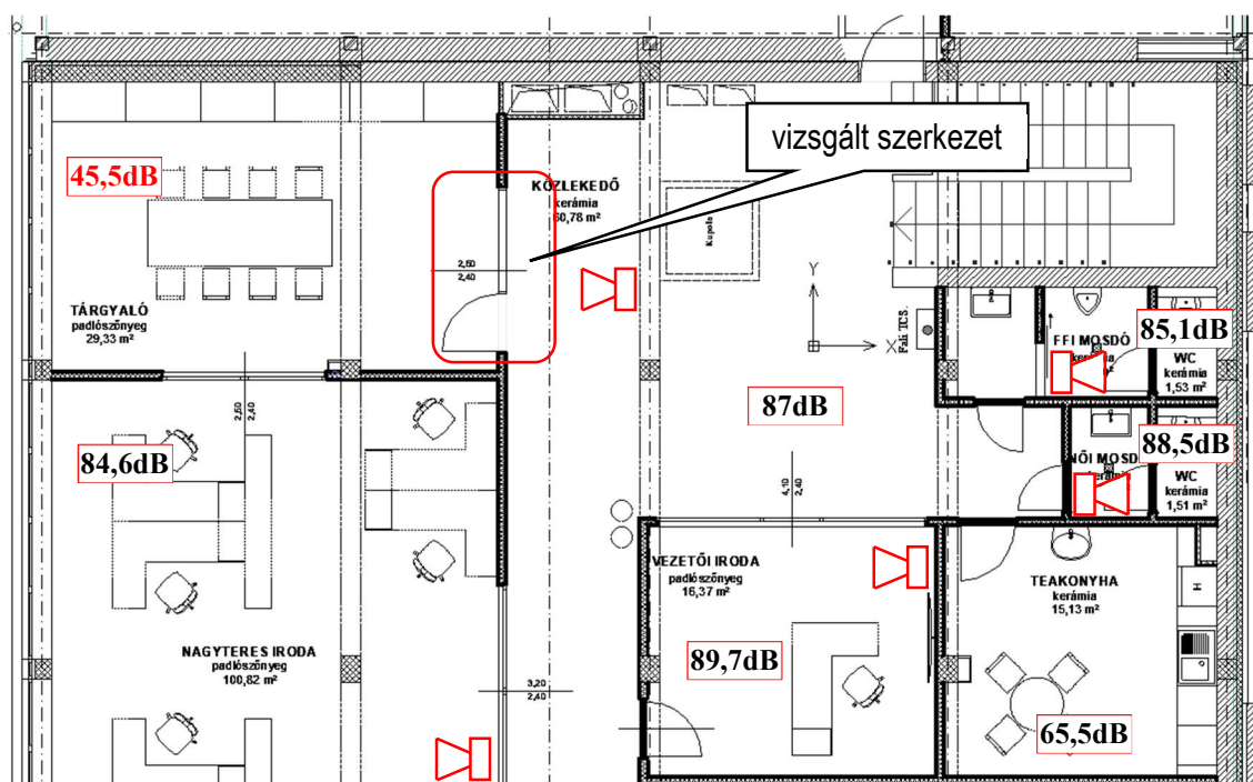
40. ábra: Hangnyomás szint mérési pontok megválasztása (részletrajz), Forrás: saját ábra
