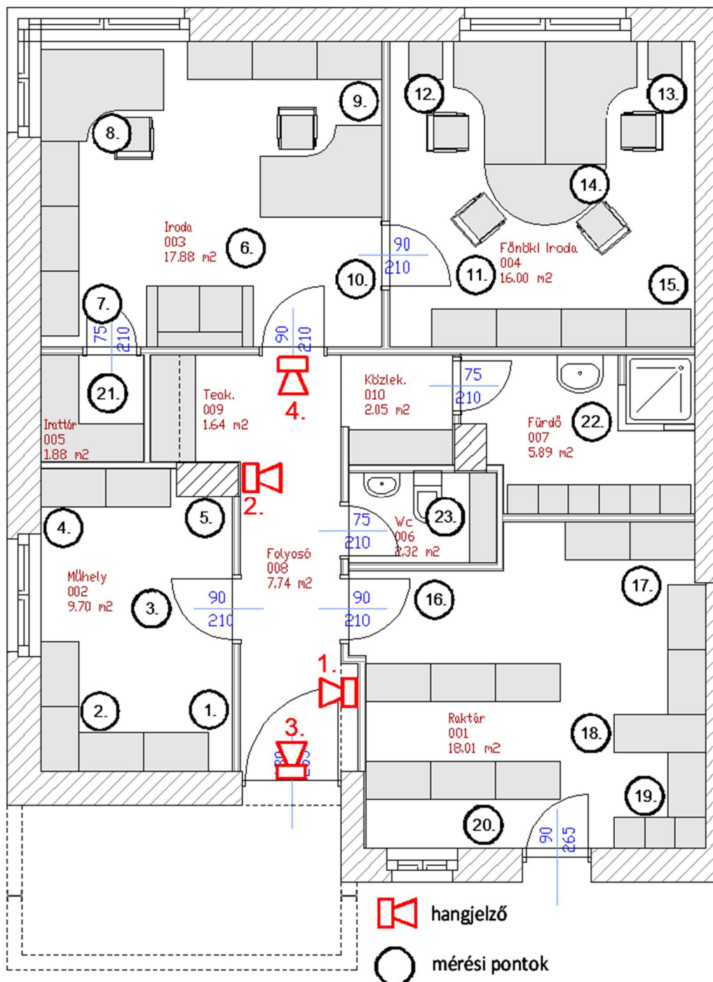
46. ábra: A Mérés 3) helyszíne, valamint a hangforrás és a mérési pontok pozíciói, forrás: saját
