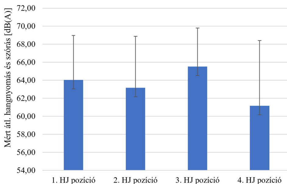
50. ábra: A Raktáron belül azonos hangjelző pozíció mellett mért hangnyomás értékek átlaga és szórása a mérési pontok alapján, forrás: saját
