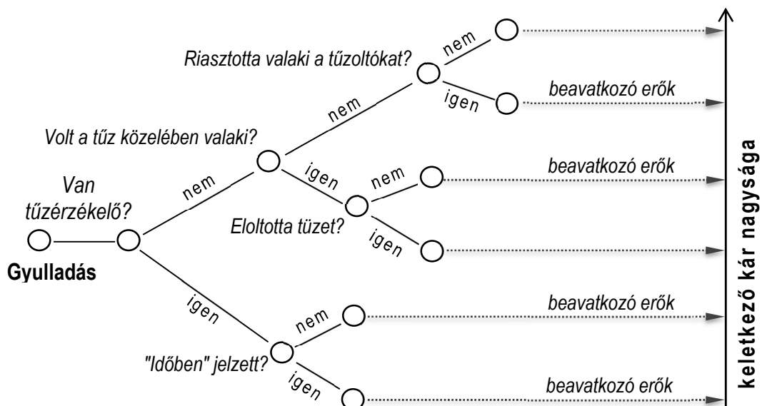
65. ábra: Eseményfa a tűz súlyossága, az észlelés és a beavatkozás függvényében [39], [10]
