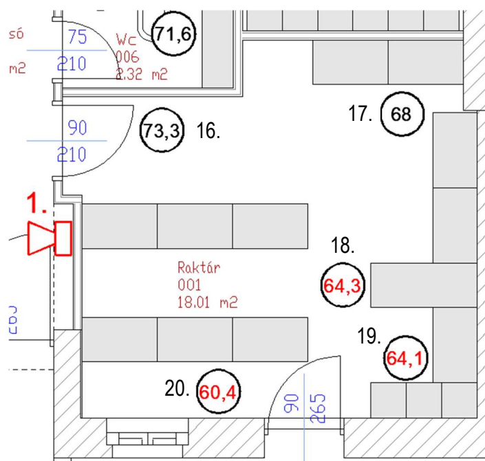
48. ábra: Az eltérő mérési pontokon mért hangnyomásszint értékek összehasonlítása a Raktárban,
