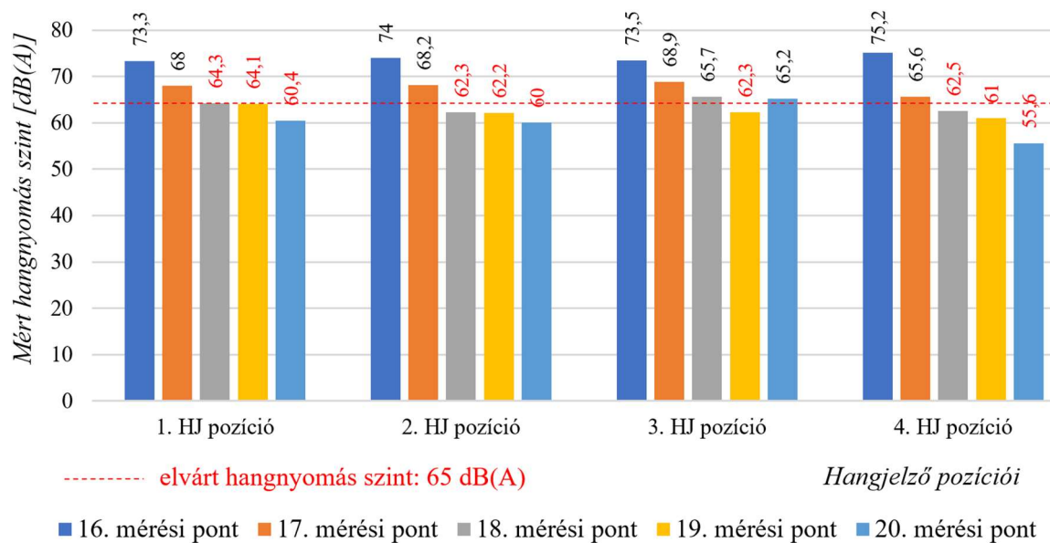
49. ábra: A Raktáron belül azonos hangjelző pozíciók esetén a mérési pont megváltoztatásának hatása a mért hangnyomás értékekre, forrás: saját
