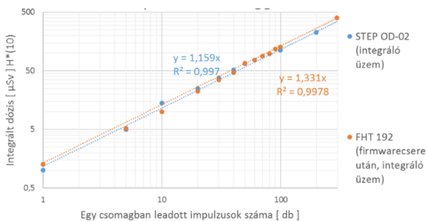
71. ábra: A csomagokban leadott dózisértékek a második körös összehasonlításban, az FHT 192 ionkamra adatgyűjtőjének firmware cseréje után integráló üzemű mérésben [19] A több mérésre vonatkoztatott, egy impulzusra jutó dózist úgy kaptam meg, hogy az egyes csomagmérések dózisait elosztottam az impulzusszámaikkal, majd átlagot számoltam. Ez STEP OD-02 esetében 1,20 \mu\text{Sv}/\text{impulzus} 11,1 %-os relatív szórással; FHT 192 esetében 1,22 \mu\text{Sv}/\text{impulzus} 9,2 %-os relatív szórással. Azaz szórásaikon belül jól megegyeznek az eredmények. Az FHT 192 esetében az átlag és a relatív szórás értéke jól visszaadja, hogy
