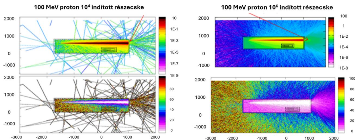
49. ábra: 100 MeV energiájú protonnyalábtól származó dózistér szimulációja, oldalnézet (felül fajlagos dózis, alul a szórás) százezer (felső), illetve egymillió darab (alsó) indított részecskére, x, y [cm], színekód: [fSv/részecske/1db 100 MeV proton], alsó ábra szórás [%].
