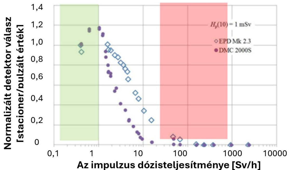
67. ábra: Állandó dózissal besugarazott EPD-k mért értékei az impulzus idő csökkenésének függvényében, zöld tartomány kvázi stacioner sugárzás, piros tartomány intenzív pulzált tér [28].
