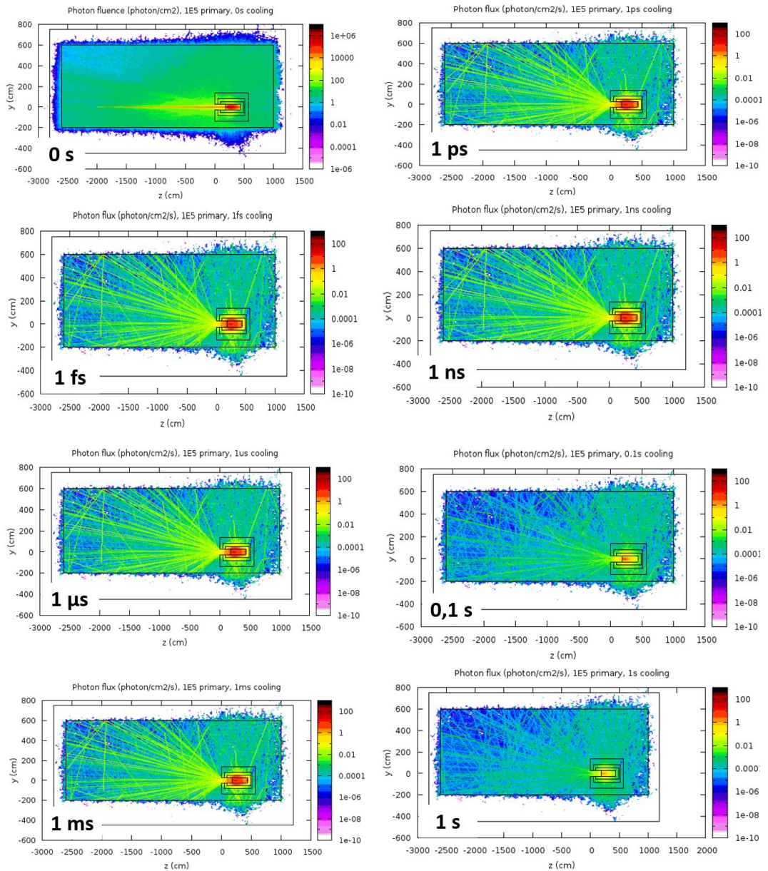
73. ábra: Foton fluens időbeli változása, FLUKA szimulációk alapján
