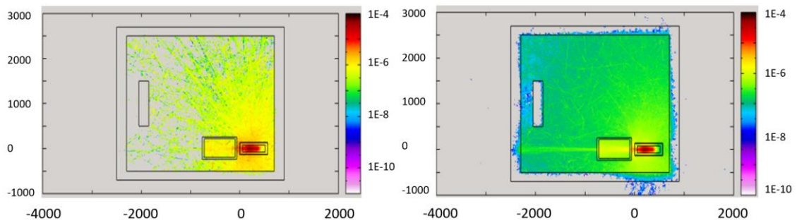
39. ábra: 2 GeV elektron nyaláb neutron fluens tere, baloldal polietilén nélkül, jobboldalt polietilén használatával, x, y [cm], színskód 10^{-4} - 10^{-16} [n/cm 2 / 1 db 2 GeV elektron]
