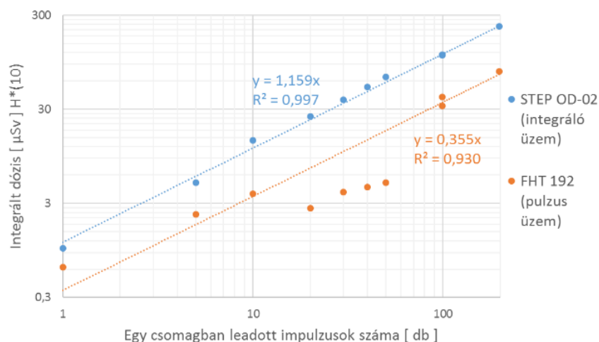
70. ábra: A csomagokban leadott dózisértékek az első tesztkörös összehasonlításban [19]
