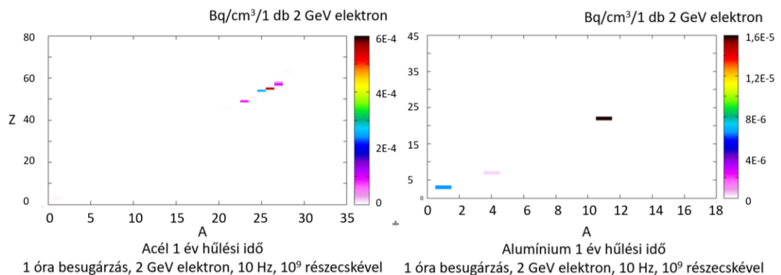
41. ábra: Acél és alumínium remanens felaktivált termékei 1 évvel a besugárzást követően, x: A, y: Z, színskód: Bq/cm 3 /1 db 2 GeV elektron
