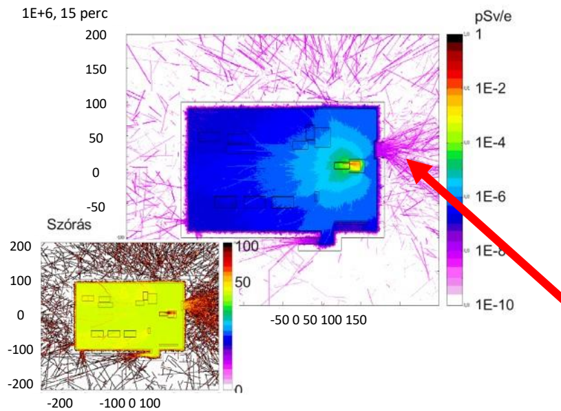
51. ábra: MTA besugárzó terem felülnézeti ábrája. Indított részecskeszám: 1 millió, futtatási idő 15 perc, alsó ábra: MTA besugárzó terem felülnézeti ábrája, a fajlagos dózis értékek szórása [%], x, y [cm], színekód: [pSv/elektron]
