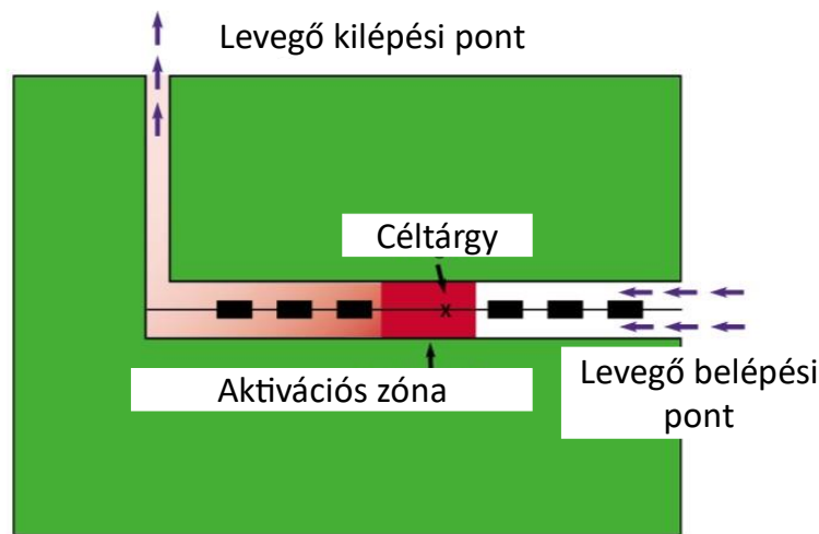
48. ábra: Lamináris áramlási modell [53]
