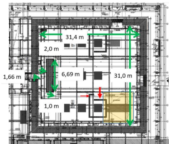
34. ábra: 2 GeV elektron nyaláb a HTA teremben
