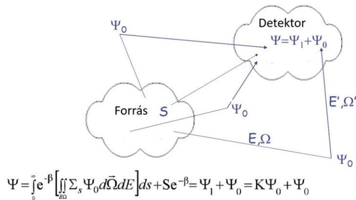
22. ábra: A FLUKA kód detektora egyszeres részecske szóródás esetén [23]
