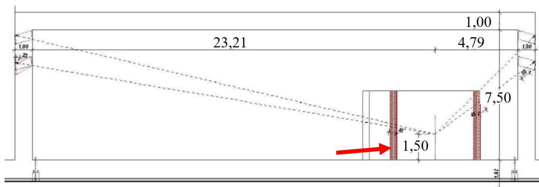
28. ábra: Az MTA besugárzó terem oldalnézete [79]
