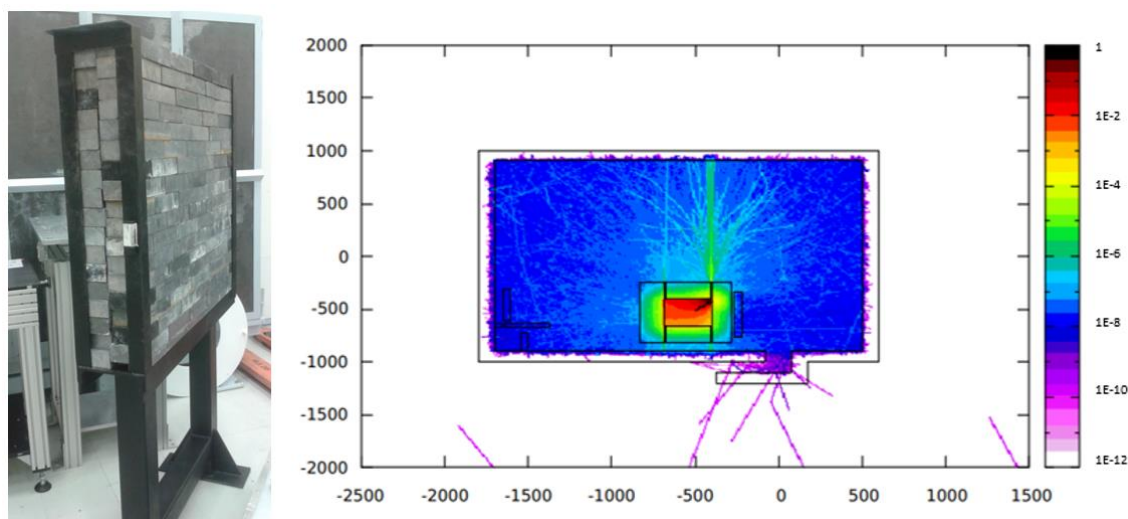
56. ábra: Baloldali ábra: árnyékoló elem, melyben a téglák nem fednek át, illetve a keret nem összeilleszthető másikkal, jobboldali ábra: besugárzó terem felülnézete, 10 MeV elektron fajlagos dózis tere. Geometriai hézag hatása a fajlagos dózis térre, x, y [cm], színskód: [pSv/elektron]
