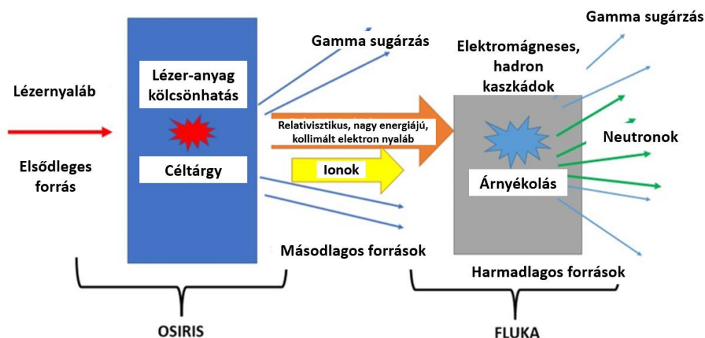
26. ábra: A lézerfény - anyag kölcsönhatás paramétereinek meghatározása és az árnyékolás (nyalábcsapda) tervezés lépései
