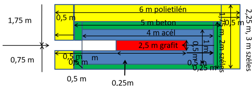
38. ábra: 2 GeV elektronnyalábhoz használt nyalábcsapda
