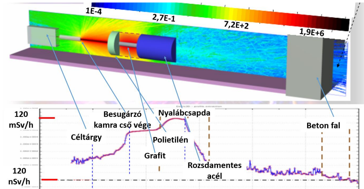
32. ábra: A csehországi nyalábcsapda és az összegzett prompt dózis alakulása [80]
