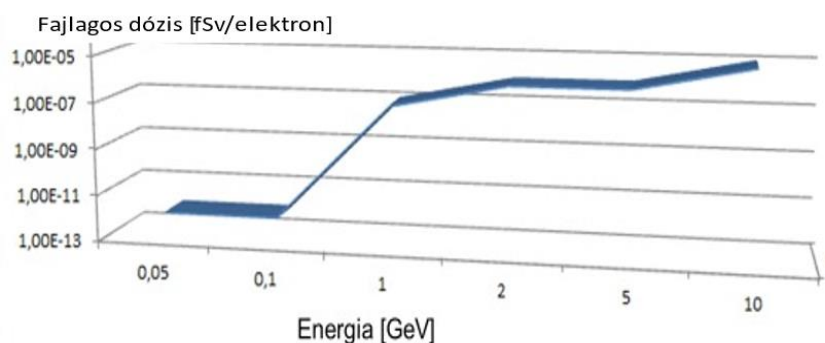
57. ábra: A növekvő elektron energia hatása a külső fajlagos dózistérre
