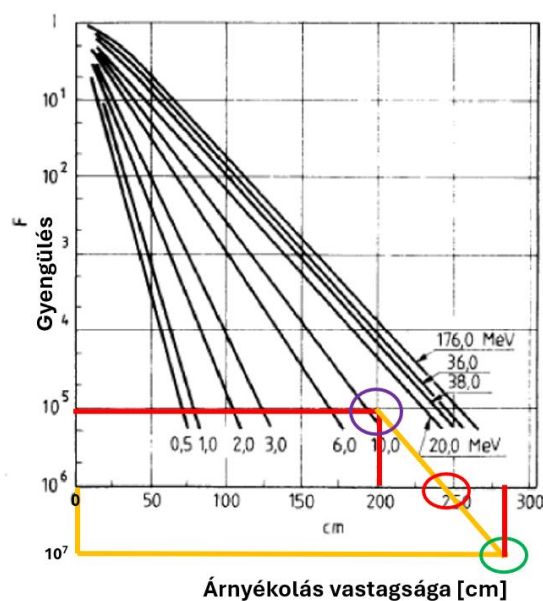
24. ábra: Fékezési röntgensugárzás széles nyalábjának gyengülése betonban [58]
