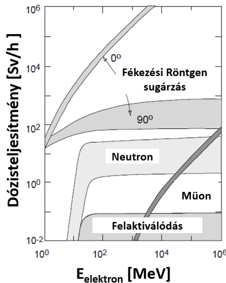
14. ábra: Az 1 MeV-1 TeV között lejátszódó folyamatok [22]
