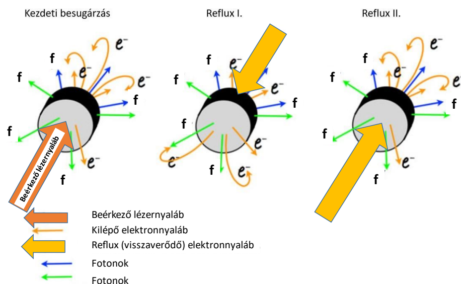
17. ábra: A céltárgyban kialakuló elektron reflux folyamata [117]
