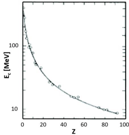
13. ábra: A kritikus energia változása a rendszám függvényében [22]
