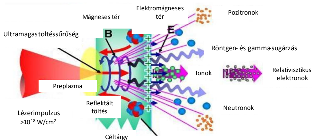
4. ábra: A lézerfény - anyag kölcsönhatása során keltett részecskék [50]
