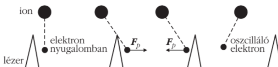
8. ábra: A lebegő hullám előállítása [44]
