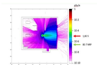
3. FLUKA szimuláció
