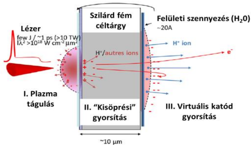
10. ábra: A TNSA kölcsönhatás folyamata [51]
