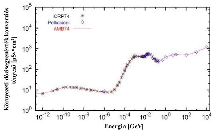
21. ábra: A FLUKA kód ICRP 74 ajánlás alapján meghatározott konverziós koefficiens függvénye (AMB74) [23]
