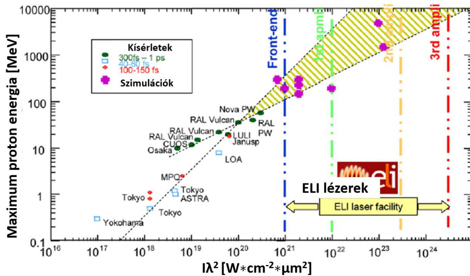
11. ábra: Maximális proton nyaláb energia a lézerfény intenzitásának függvényében [51]
