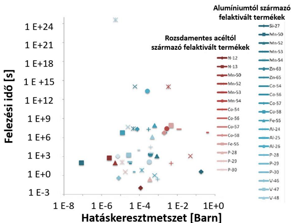
47. ábra: Alumínium és rozsdamentes acélban keletkező felaktivált radionuklidok felezési ideje a hatáskeresztmetszet függvényében, 1 barn= 10^{-28} m 2 [39]
