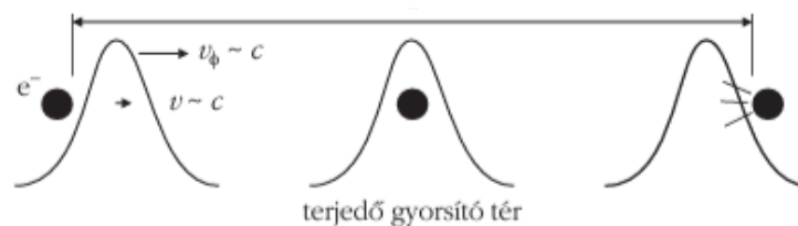
5. ábra: Plazmahullám alapú részecskegyorsítás [44]
