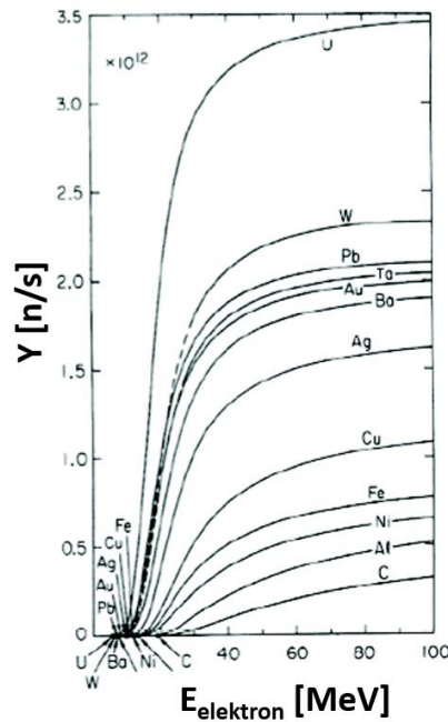
15. ábra: Óriás rezonancia neutron hozam az elektron energia függvényében [22]
