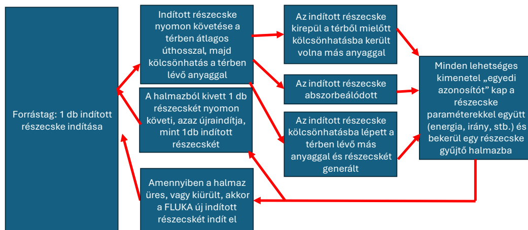
23. ábra: Egy indított részecske nyomon követése a FLUKA kódban [23]
