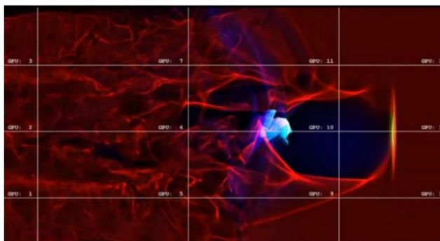
9. ábra: A buborék gyorsítás szimulációja, az elektronsűrűség a sötétebb árnyalatok felé csökken [46]
