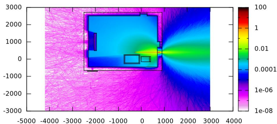
35. ábra: 2 GeV elektron nyaláb fajlagos dózis tere a HTA teremben
