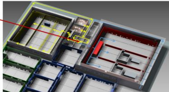
61. ábra: Az ELI ALPS dozimetriai rendszere
