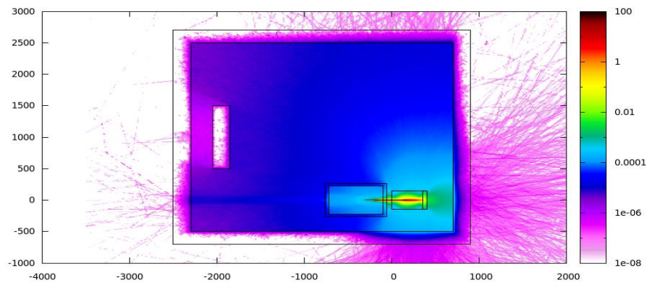
40. ábra: 2 GeV elektron nyaláb fajlagos dózis tere a HTA teremben, rozsdamentes acél helyett alumíniumot használva, színskód [fSv/1 db 2 GeV elektron] nyalábcsapda alkalmazásával, x, y [cm]
