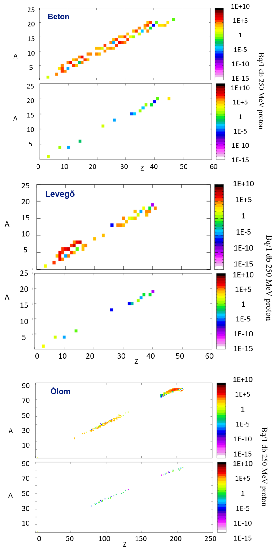
45. ábra: Különféle anyagok felaktiválódása
