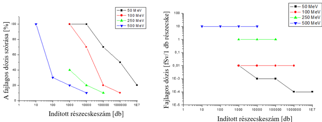
50. ábra: 50-500 MeV energiájú protonok által generált fajlagos dózistér és szórás értékek a sugárvédelmi fal külső felületén az indított részecskeszám függvényében, x, y [cm], színkód: [fSv/részecske], szórás [%]
