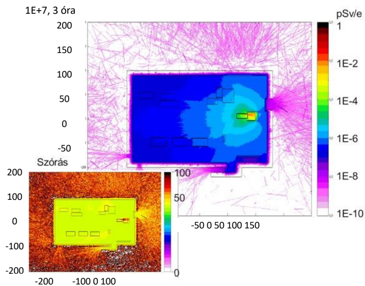
52. ábra: MTA besugárzó terem felülnézeti ábrája. Indított részecskeszám: 10 millió, futtatási idő 3 óra, alsó ábra: Besugárzó terem felülnézeti ábrája. a fajlagos dózis értékek szórása [%], x, y [cm], színekód: [pSv/elektron]
