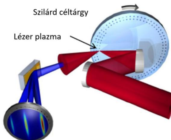
16. ábra: Szilárd céltárgy besugárzása [100]
