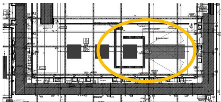
25. ábra: A HTA SPWe besugárzó kamra körüli lokális árnyékolás [79]
