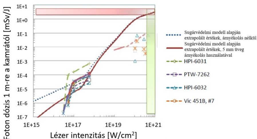
18. ábra: 10^{21} \text{ W/cm}^2 lézer intenzitásnál várhatóan kialakuló fajlagos röntgen foton dózisterek értéke a SLAC-ban üzemelő besugárzó kamra körül [11]
