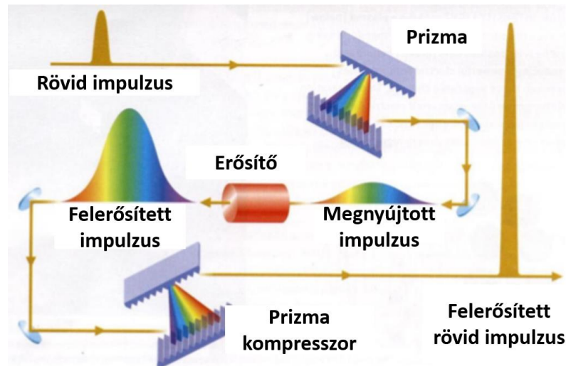
2. ábra: A CPA elven működő lézernyaláb erősítés [40]
