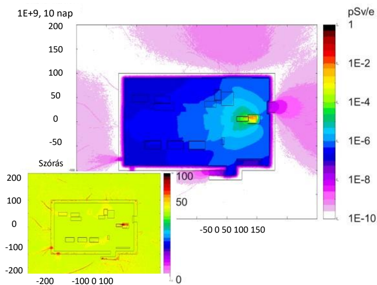
54. ábra: MTA besugárzó terem felülnézeti ábrája. Indított részecskeszám: 1000 millió indított részecskével, futtatási idő 10 nap, alsó ábra: Besugárzó terem felülnézeti ábrája. a fajlagos dózis értékek szórása [%], x, y [cm], színekód: [pSv/elektron]
