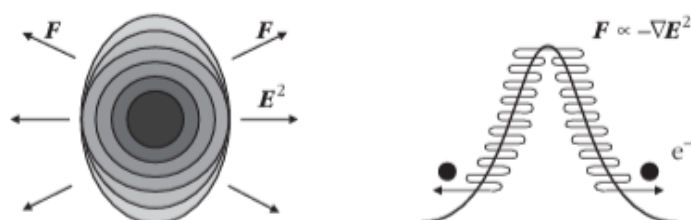
6. ábra: A ponderomotoros erő gyorsítása [44]
