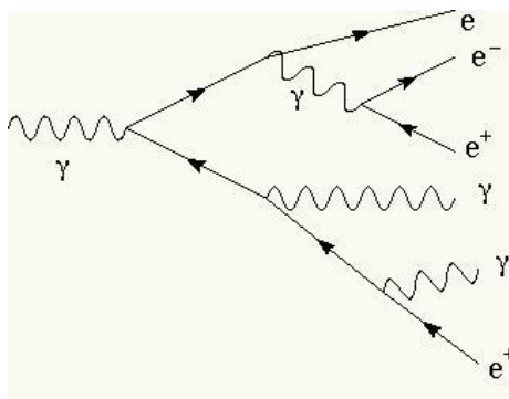
12. ábra: Elektromágneses kaszkád effektus, [114]
