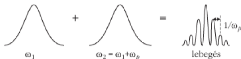
7. ábra: A lebegő hullám előállítása [44]
