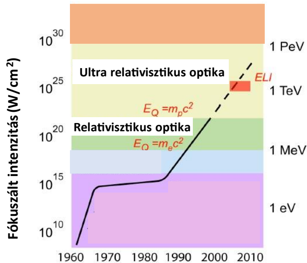
3. ábra: A lézerek fókuszált intenzitásának növekedése 1960-tól napjainkig [48]
