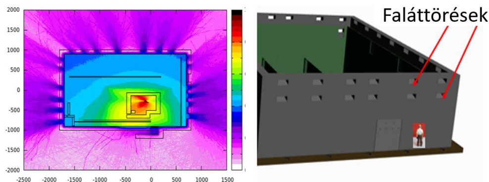
29. ábra: A felső faláttöréseken kiszóródó sugárzások
