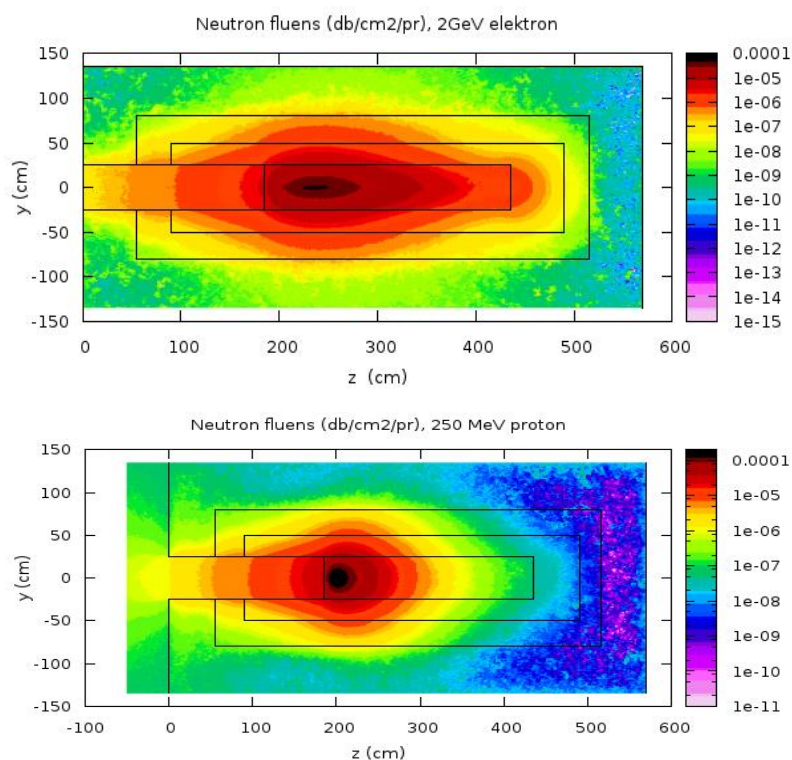
46. ábra: Az elektromágneses- és hadronkaszád által generált neutron fluens a HF PW nyaláb csapdában [91]
