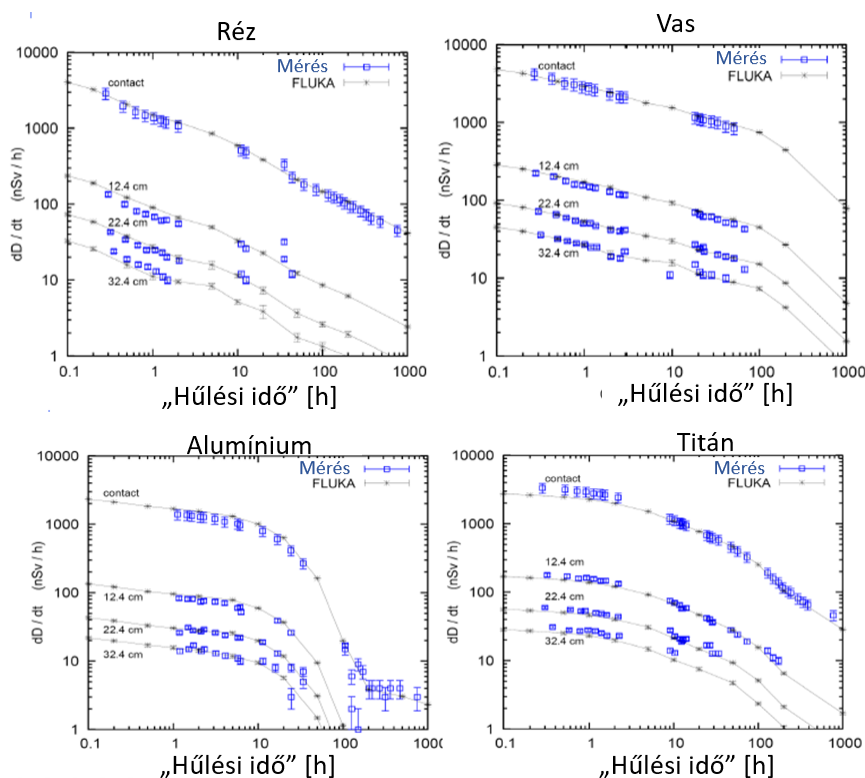
19. ábra: A FLUKA kód által számított remanens dózisteljesítmények összevetve műszeres mérésekkel [76]
