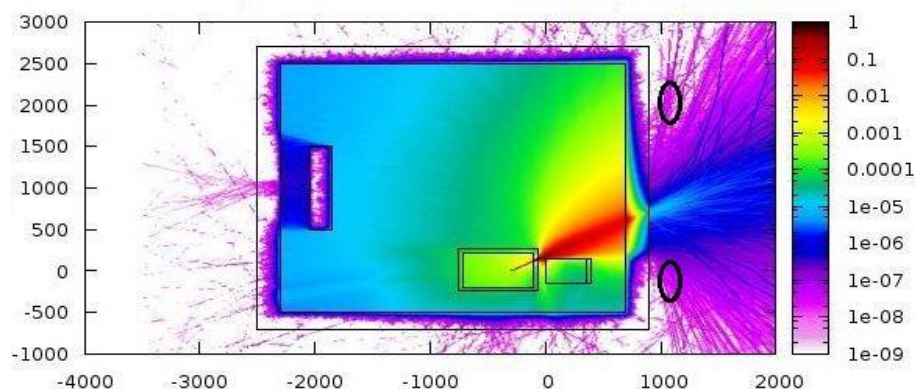
36. ábra: 2 GeV elektron nyaláb fajlagos dózis tere a HTA teremben
