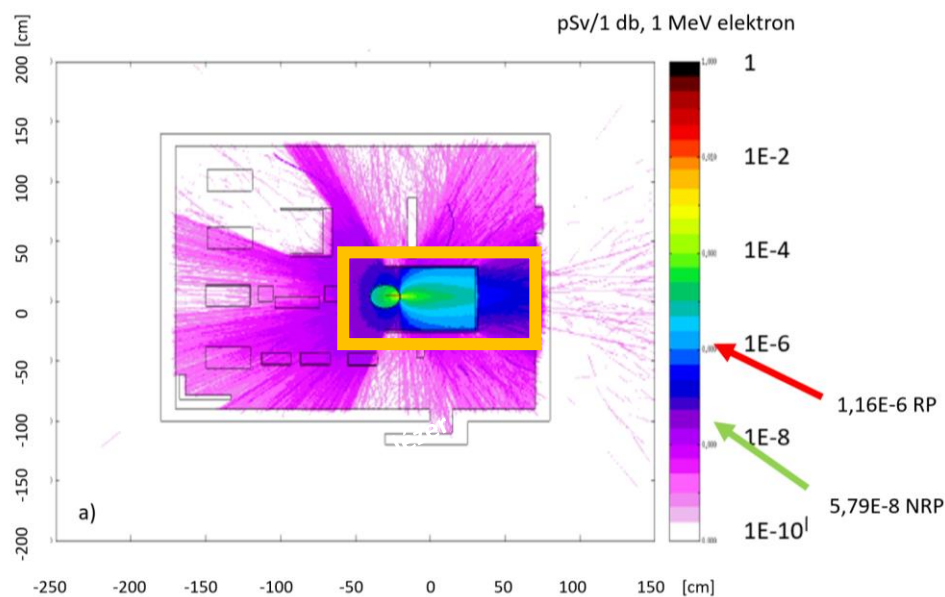
59. ábra: A LEIA berendezés fajlagos dózis terének felülnézeti térképe, jelölve a „sugárveszélyes munkaköri besorolású” (RP) és „nem sugárveszélyes munkaköri besorolású” (NRP) munkavállalói fajlagos dózis limit szinteket, x, y [cm], színkód: [pSv/1 MeV elektron]
