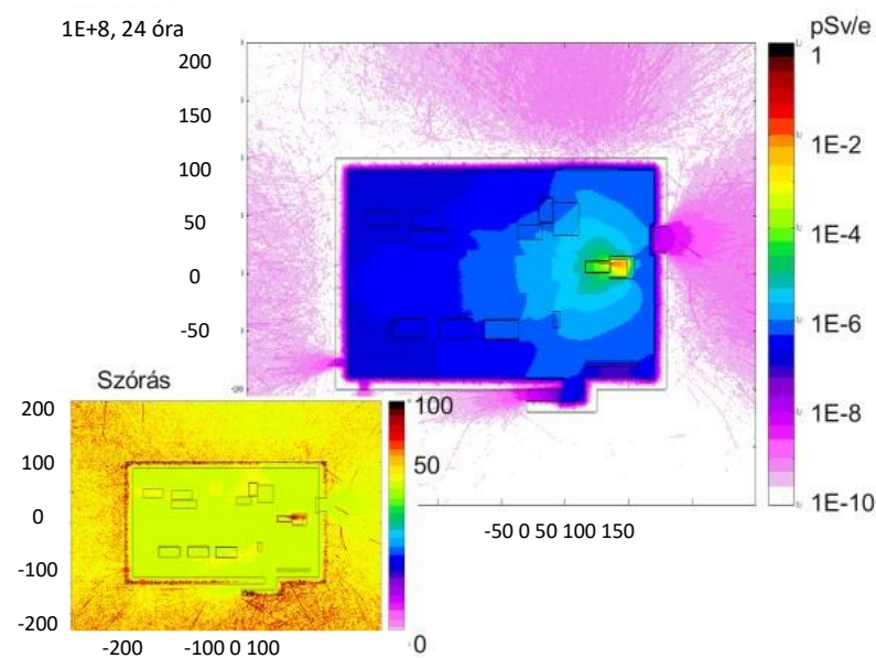
53. ábra: MTA besugárzó terem felülnézeti ábrája. Indított részecskeszám: 100 millió indított részecskével, futtatási idő 24 óra, alsó ábra: Besugárzó terem felülnézeti ábrája. a fajlagos dózis értékek szórása [%], x, y [cm], színekód: [pSv/elektron]
