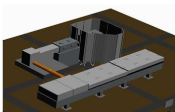
4. Optimális árnyékolás tervezet koncepcionális 3D vázlata
