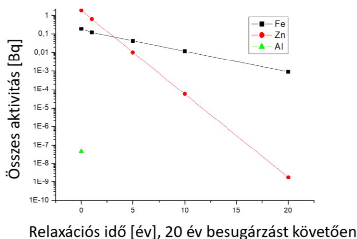
44. ábra: Összaktivitás a relaxációs idő függvényében
