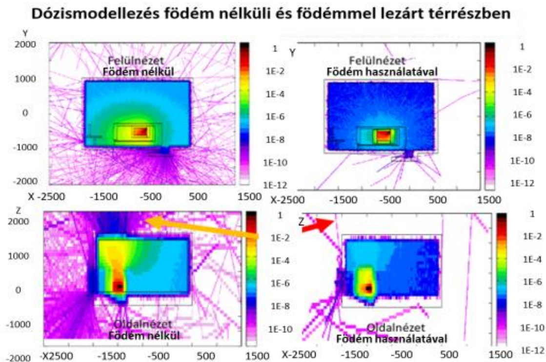
55. ábra: 10 MeV-es elektronsugárzás fajlagos dóziseloszlása. x, y, z [cm], színekód: [pSv/elektron]
