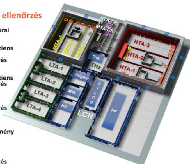
68. ábra: Az ELI ALPS „A” épület laboratóriumai és dózisteljesítmény mérő pontjai
