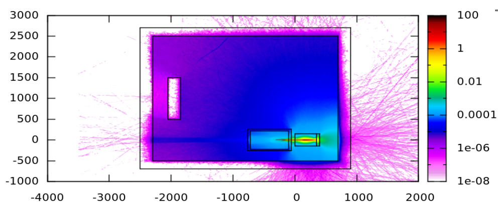
37. ábra: 2 GeV elektron nyaláb összegzett fajlagos dózis tere a HTA teremben
