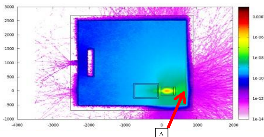
42. ábra: Várható neutron fluens ( [\text{n/cm}^2/1 \text{ db } 2 \text{ GeV elektron}] ) a HTA-ban, x, y [cm]
