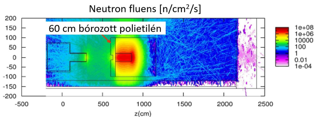
31. ábra: A nyalábcsapda továbbfejlesztett változata, bórozott polietilén ablakkal kiegészítve [81]
