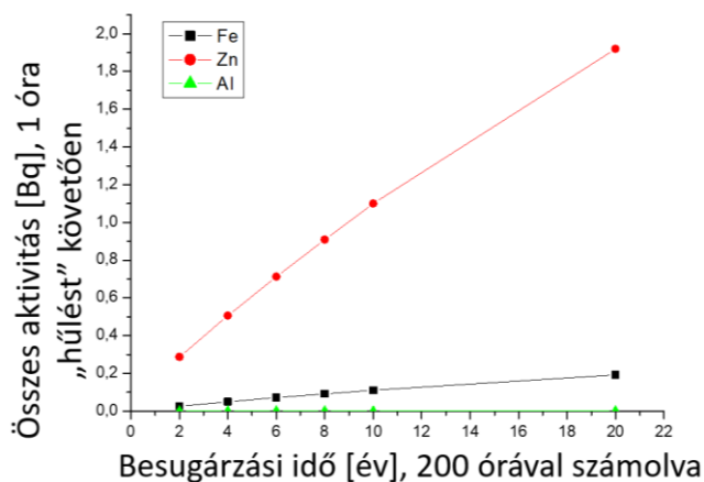
43. ábra: A Zn, Fe és Al izotópok feldúsulása az üzemelés során
