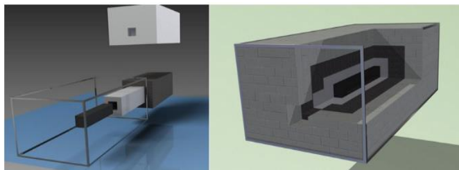
33. ábra: Különböző téglatestekből felépített nyalábcsapda
