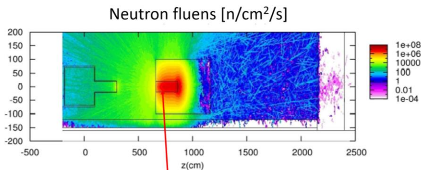
30. ábra: A nyalábcsapda továbbfejlesztett változata, grafitrúddal közepén (piros nyíl) [81]
