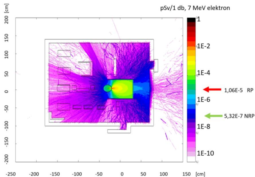
60. ábra: A LEIA berendezés fajlagos dózis terének felülnézeti térképe, jelölve a „sugárveszélyes munkaköri besorolású” és „nem sugárveszélyes munkaköri besorolású” munkavállalói fajlagos dózis limit szinteket, x, y [cm], színkód: [pSv/7 MeV elektron] A tervezés során az üzemviteli paraméter (F, T, G), vagy részecskeszám (N) változására igen érzékeny fajlagos dózist számítottam ki. A kapott értékből azonnal látható, hogy az adott meglévő árnyékolást át kell-e tervezni, ki kell-e egészíteni, és ha igen, akkor milyen mértékben.
