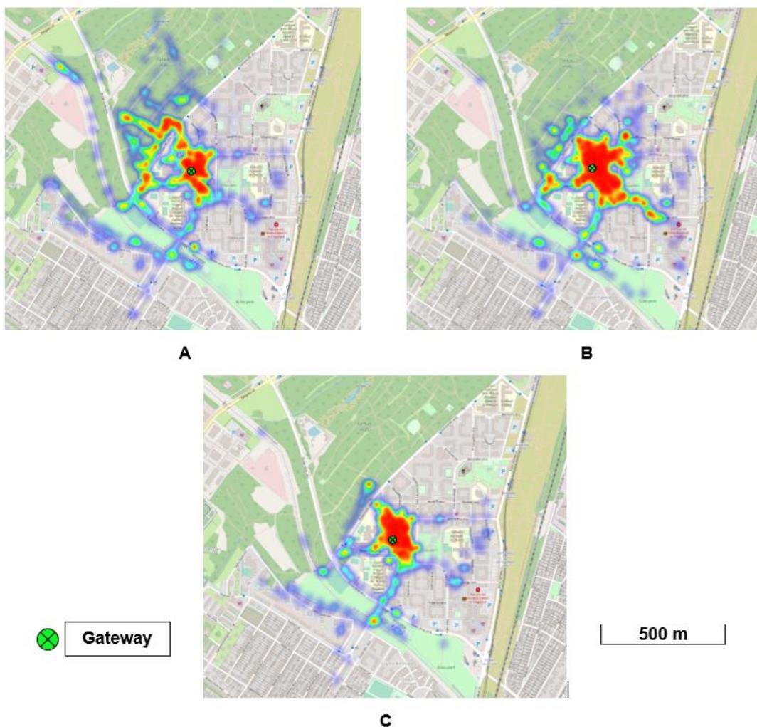
8. ábra - Mikrotik Gateway (A), Tracknet Gateway (B) és Kerlink Gateway (C) hő térképe (Készítette a szerző: [112])
