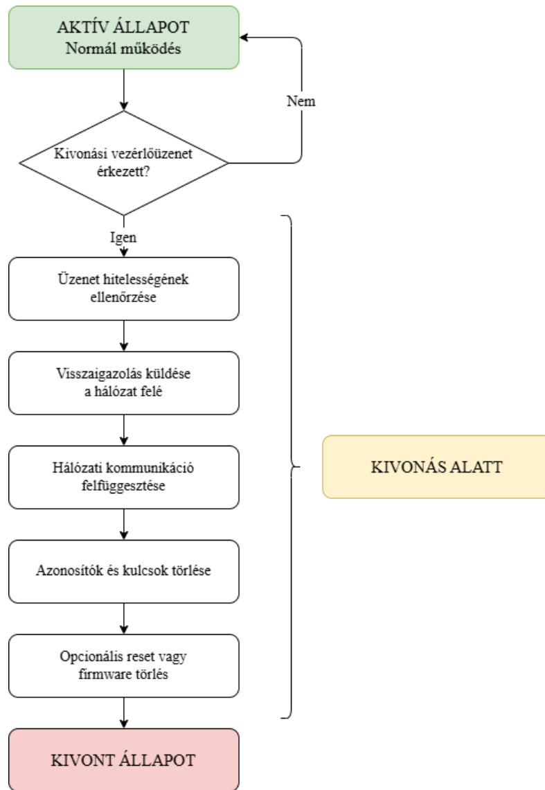
17. ábra - A kivonási eljárás végberendezés-oldali folyamata normál működés mellett (saját szerkesztés)
