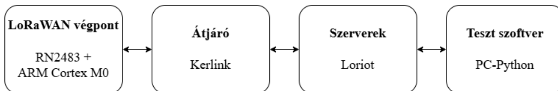
13. ábra - Képküldés mérési összeállítása (Készítette a szerző: [71])
