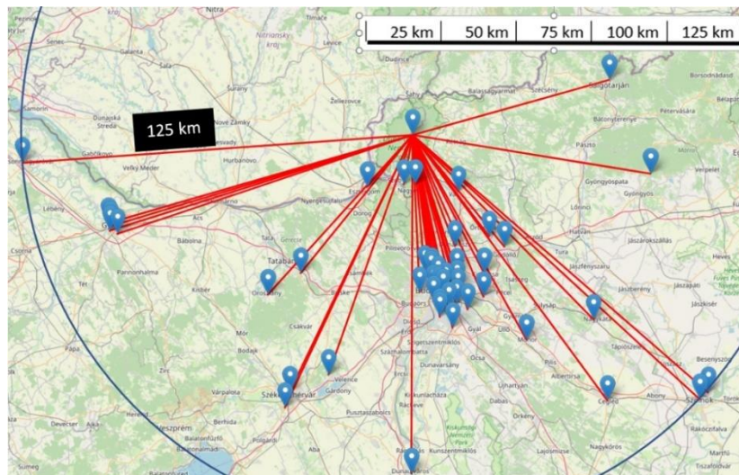
11. ábra - Mérés Csóványoson (Készítette a szerző: [103])
